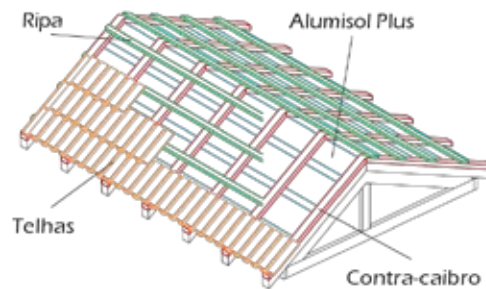
Instalação em telhados com telhas de barro ou concreto
