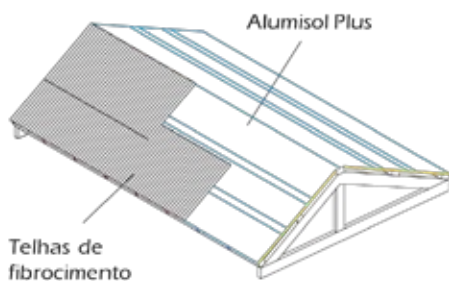
Instalação em telhados com telhas de fibrocimento
