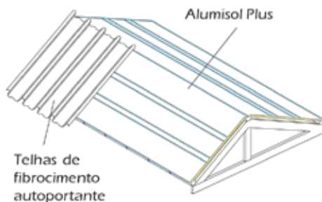
Instalação em telhados com telhas de fibrocimento autoportantes
