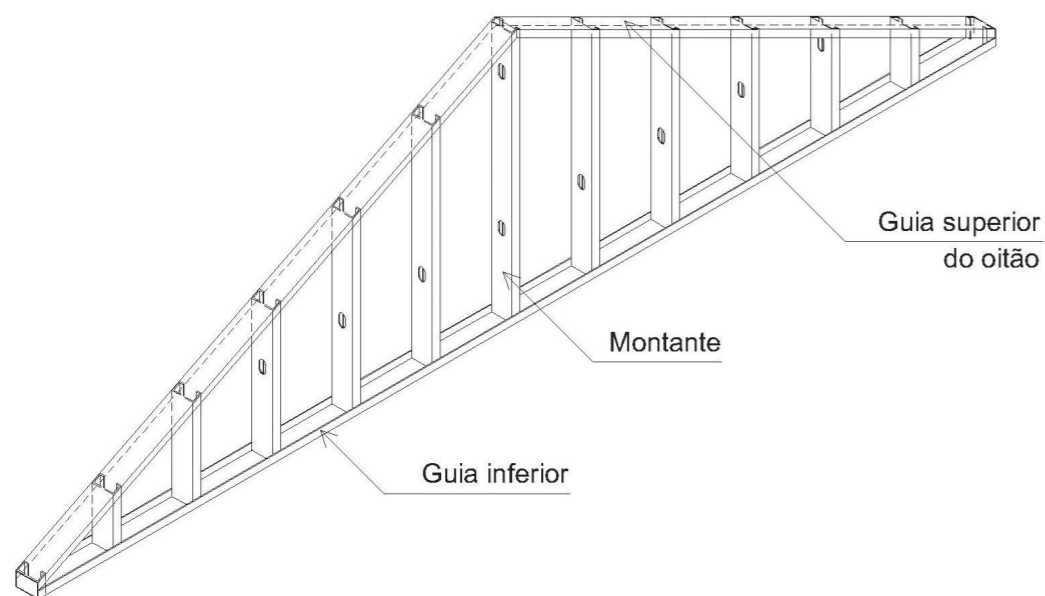
Figura 5.19 - Painel de fechamento do oitão
