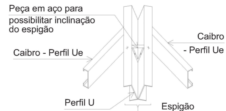
Figura 5.8 - Espigão formado a partir de dois perfis U
