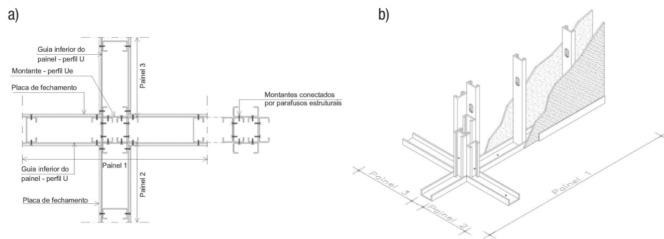
Figura 3.19 - Encontro de três painéis: a) planta b) perspectiva
