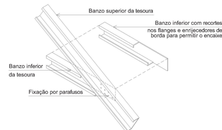
Figura 5.15 - Detalhe da união do banzo superior e inferior de uma tesoura
