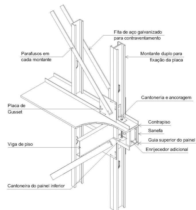
Figura 3.11 - Ancoragem de painel superior
