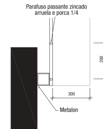
DETALHE 2
