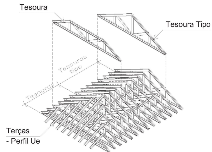
Figura 5.24 - Tesouras auxiliares
