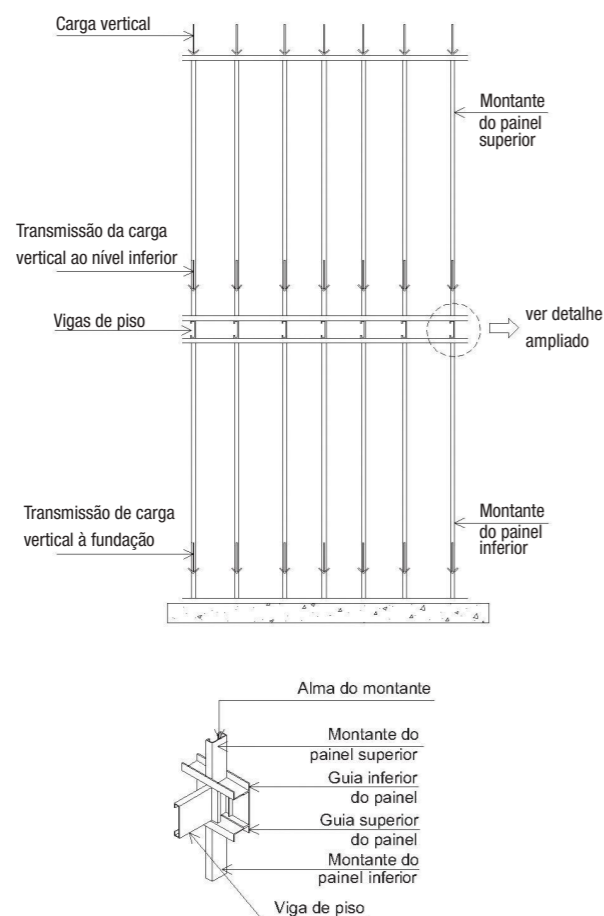
Figura 3.1 - Transmissão da carga vertical à fundação
