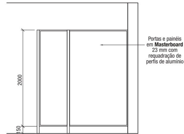
ELEVÇÃO B
