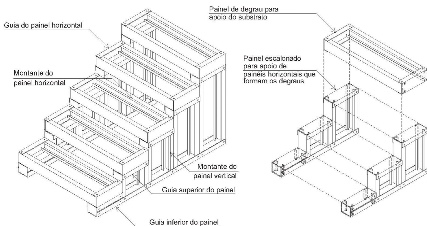
Figura 4.17 - Desenho esquemático de uma escada de painéis escalonados
