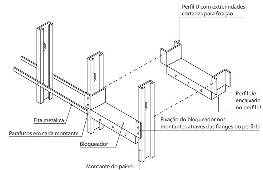
Figura 3.13 - Esquema de travamento horizontal do painel através de bloqueadores
