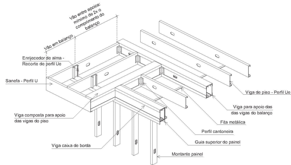
Figura 4.8 - Laje em balanço
