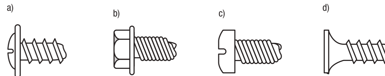
Figura 7.3 - Tipos de cabeça de parafusos mais utilizados em ligações com LSF: a) cabeça lenticular; b) sextavada; c) panela e d) trombeta.
