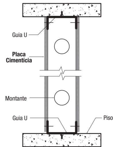
CORTE A-A FIXAÇÃO SUPERIOR E INFERIOR DA PAREDE
