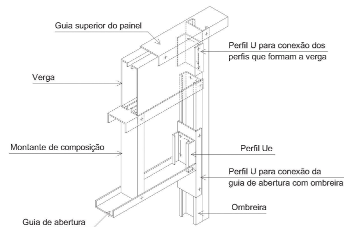
Figura 3.7 - Composição de vão de abertura
