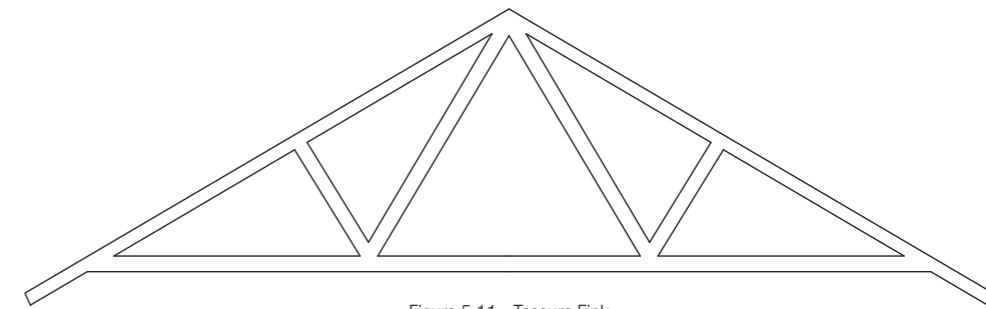
Figura 5.11 - Tesoura Fink
