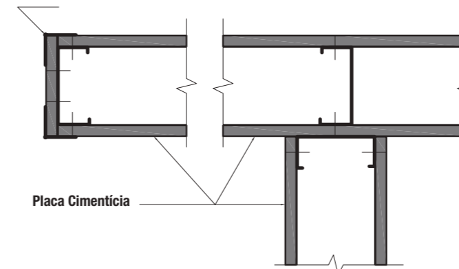
CORTE E-E ENCONTRO EM "T"
