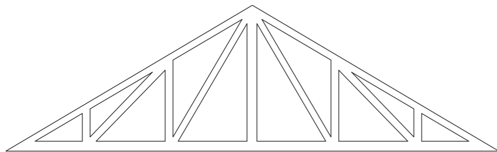
Figura 5.10 - Tesoura Pratt
