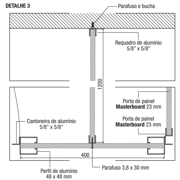
DETALHE 3
