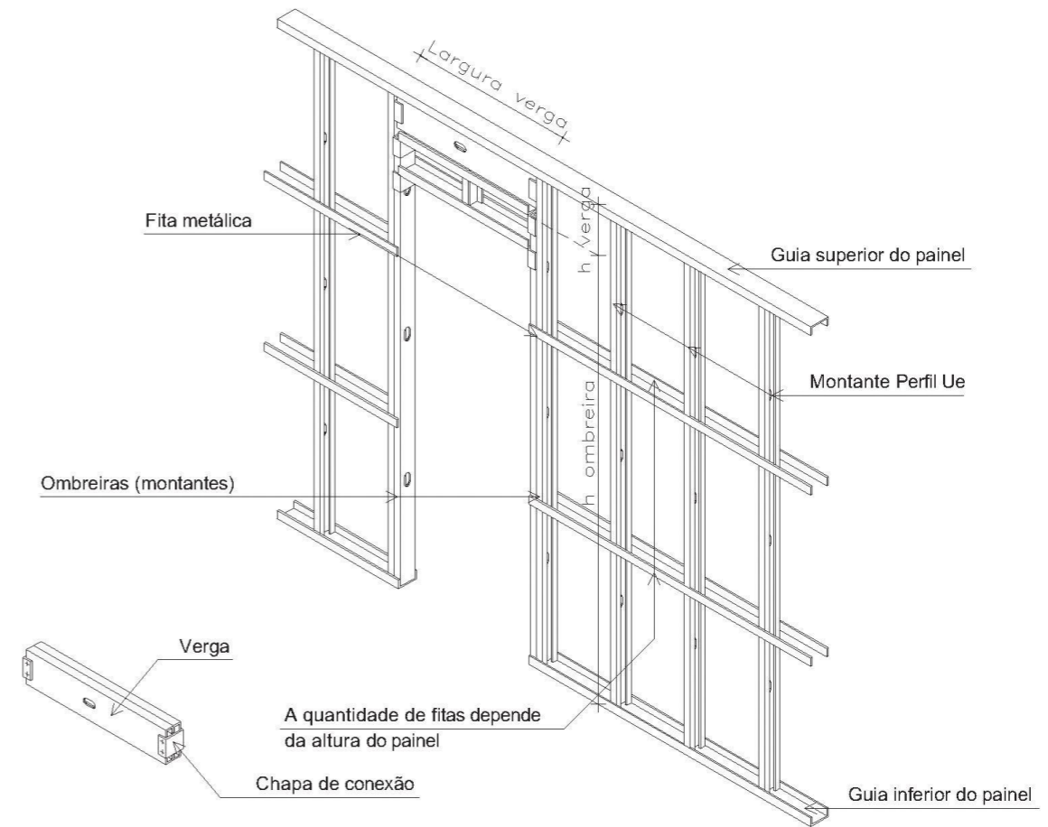
Figura 3.12 - Fita metálica para travamento de painel
