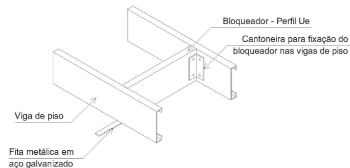
Figura 4.14 - Bloqueador
