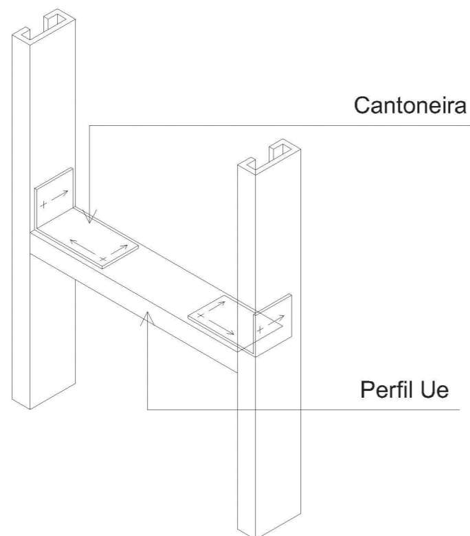
Figura 3.14 - Esquema de fixação de bloqueador através de cantoneiras
