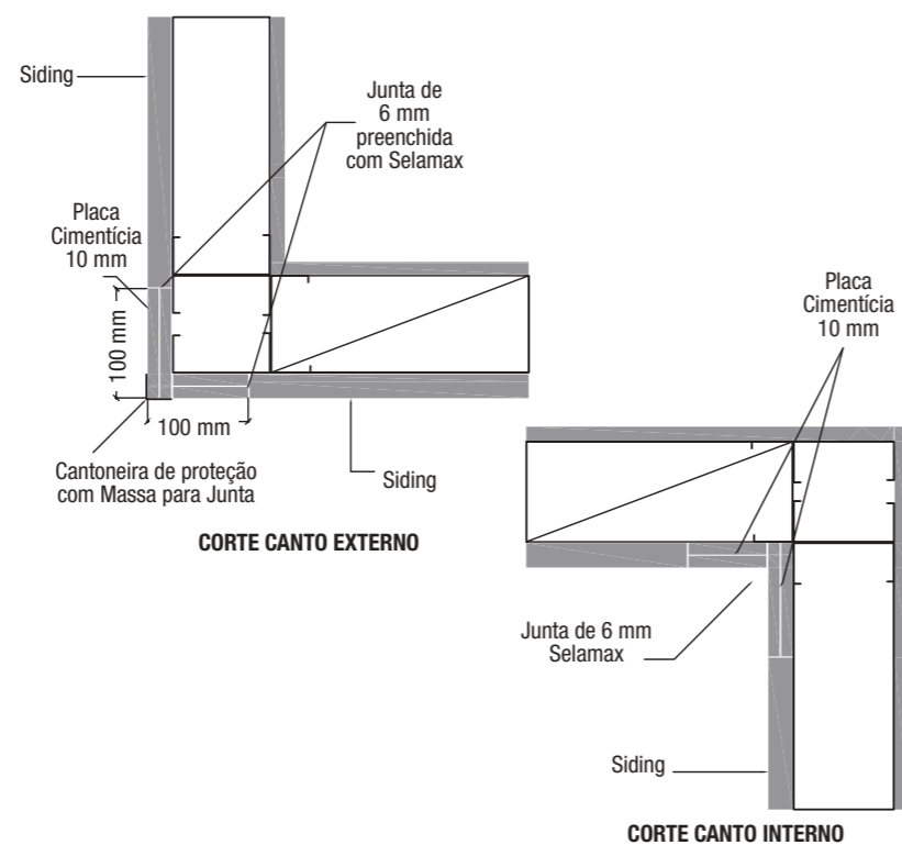
CORTE CANTO INTERNO
