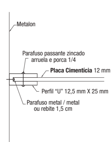
DETALHE 1
