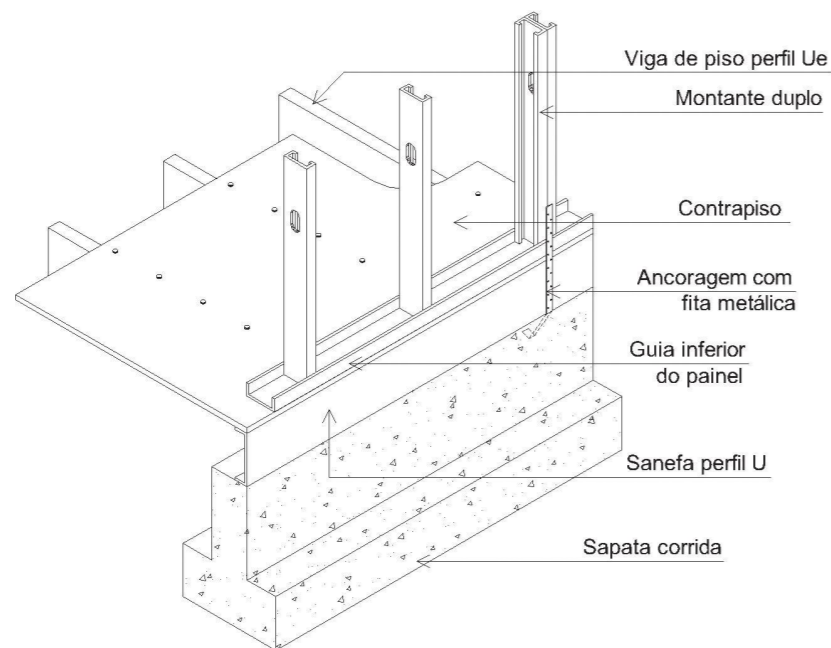
Figura 2.5 - Corte detalhado de fundação tipo sapata corrida
