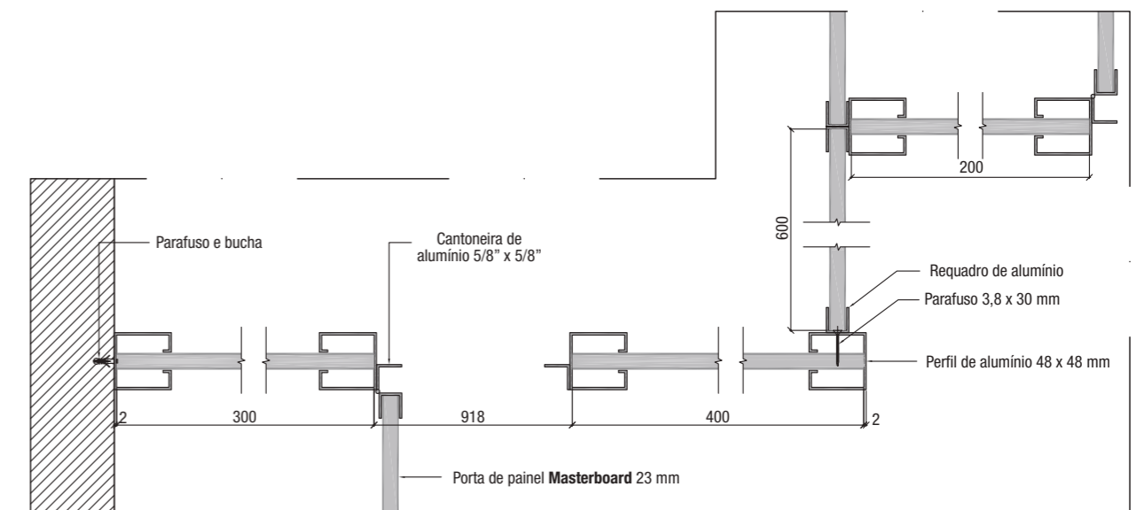
DETALHE 4
