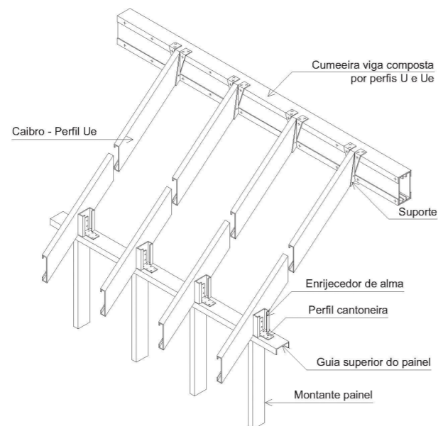
Figura 5.4 - Telhado típico estruturado com caibros
