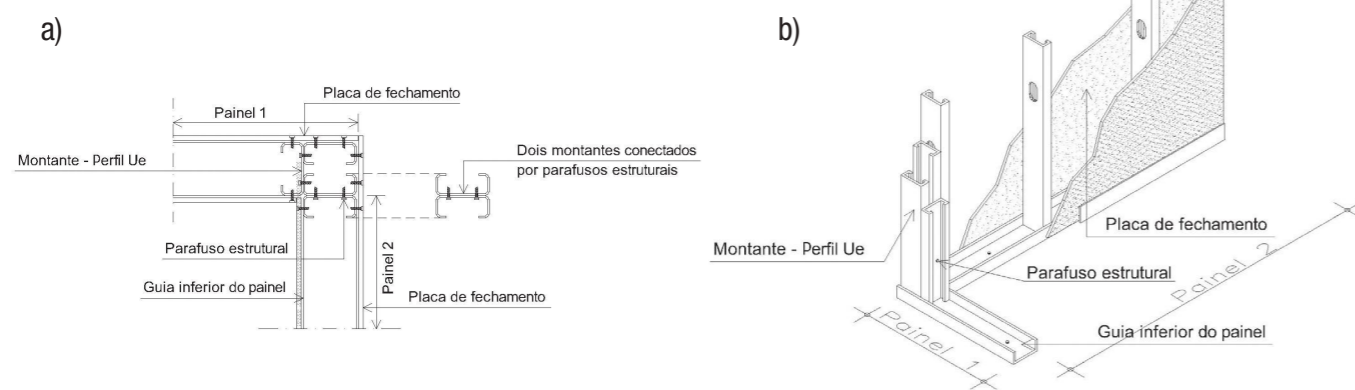
Figura 3.15 - União de dois montantes pela alma: a) planta b) perspectiva
