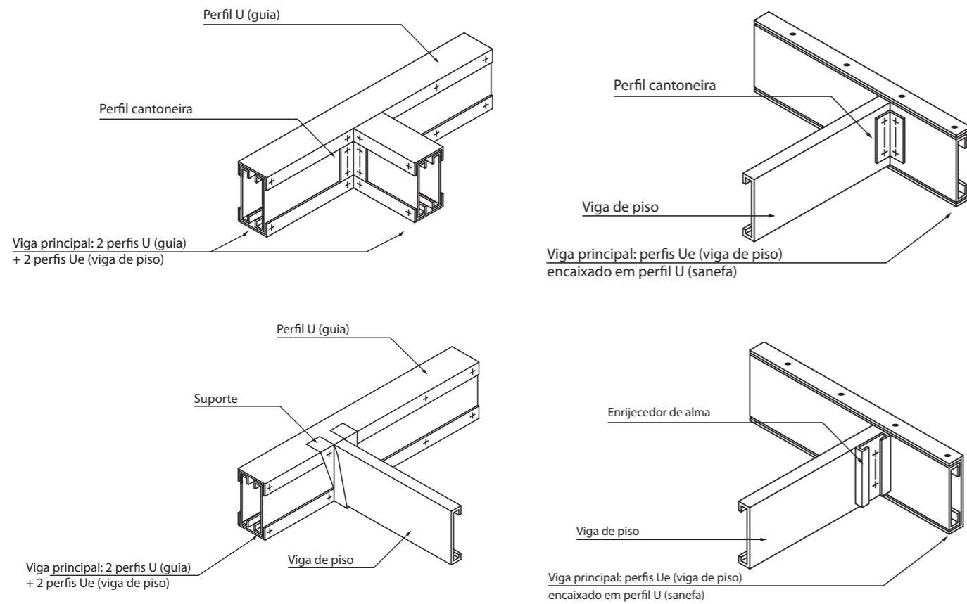
Figura 4.12 - Tipos de vigas principais para apoio de vigas de piso
