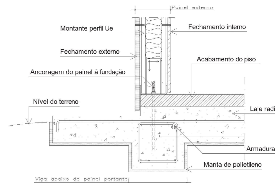
Figura 2.4 - Detalhe esquemático de ancoragem de painel estrutural a uma laje radier (adaptado de Consul Steel, 2002)
