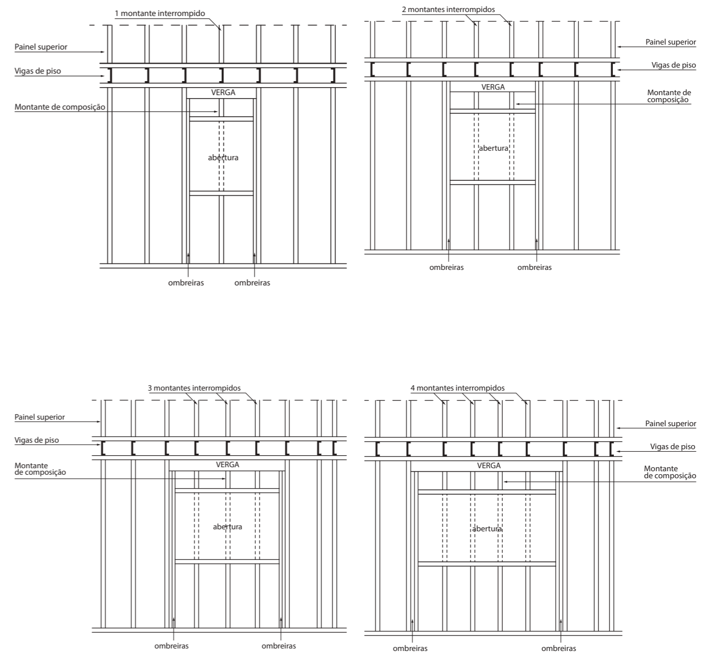
Figura 3.5 - Detalhe de ombreira
