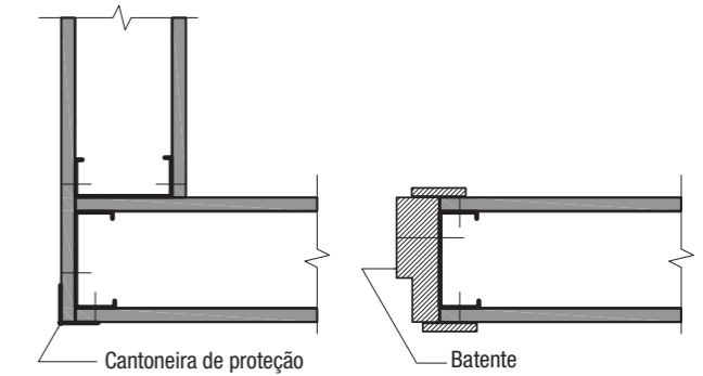
CORTE G-G FIXAÇÃO DE BATENTE
