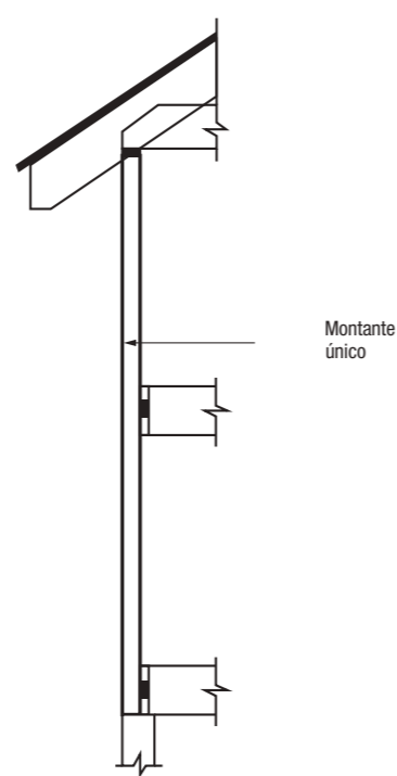
Figura 2.3 - Esquema de construção tipo “balloon” (Fonte: SCI)
