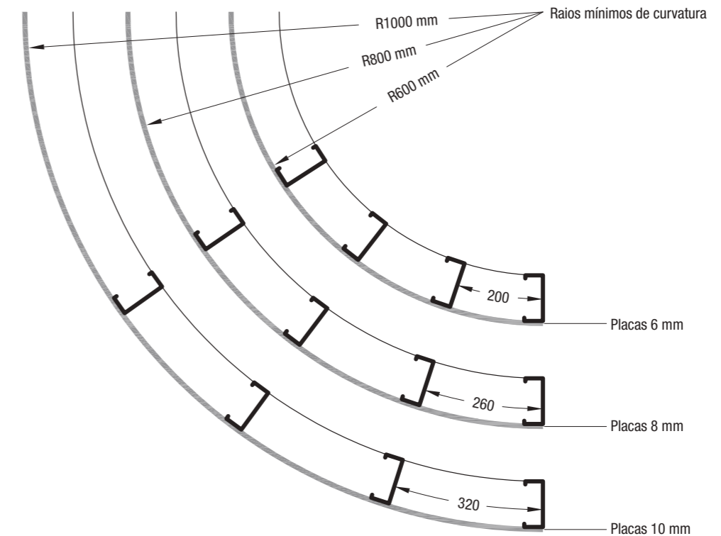
CORTE I-I PAREDES CURVAS
