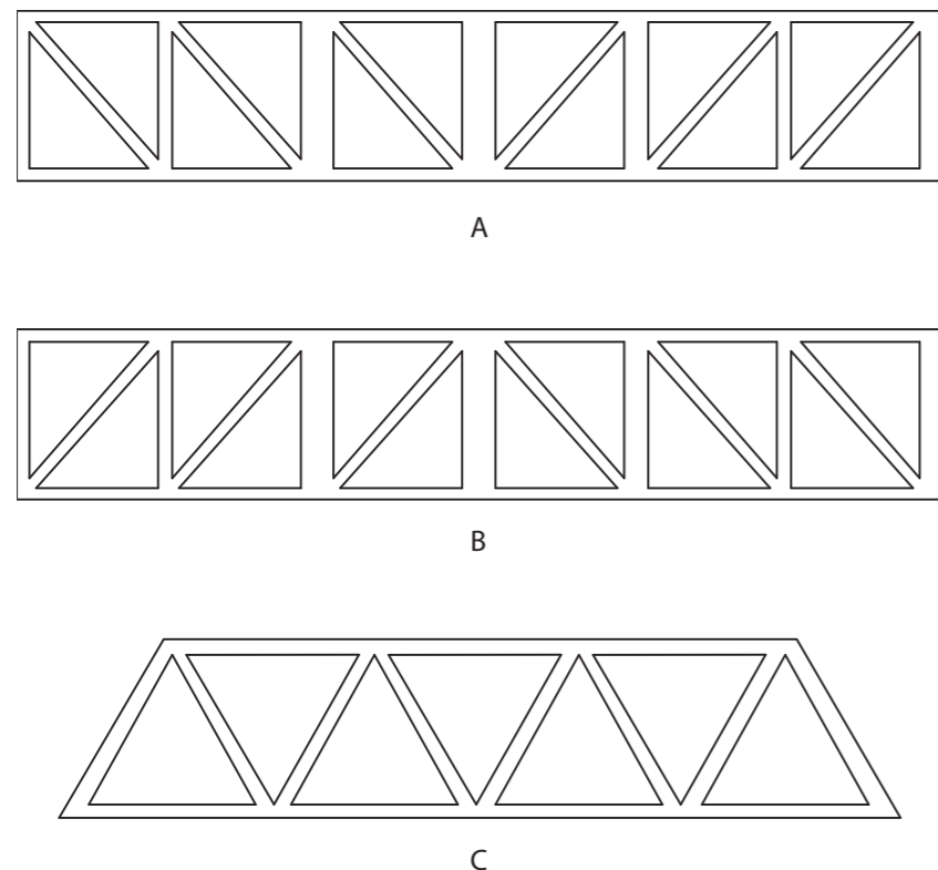
Figura 5.2 - Alguns tipos de treliças planas para Light Steel Framing
