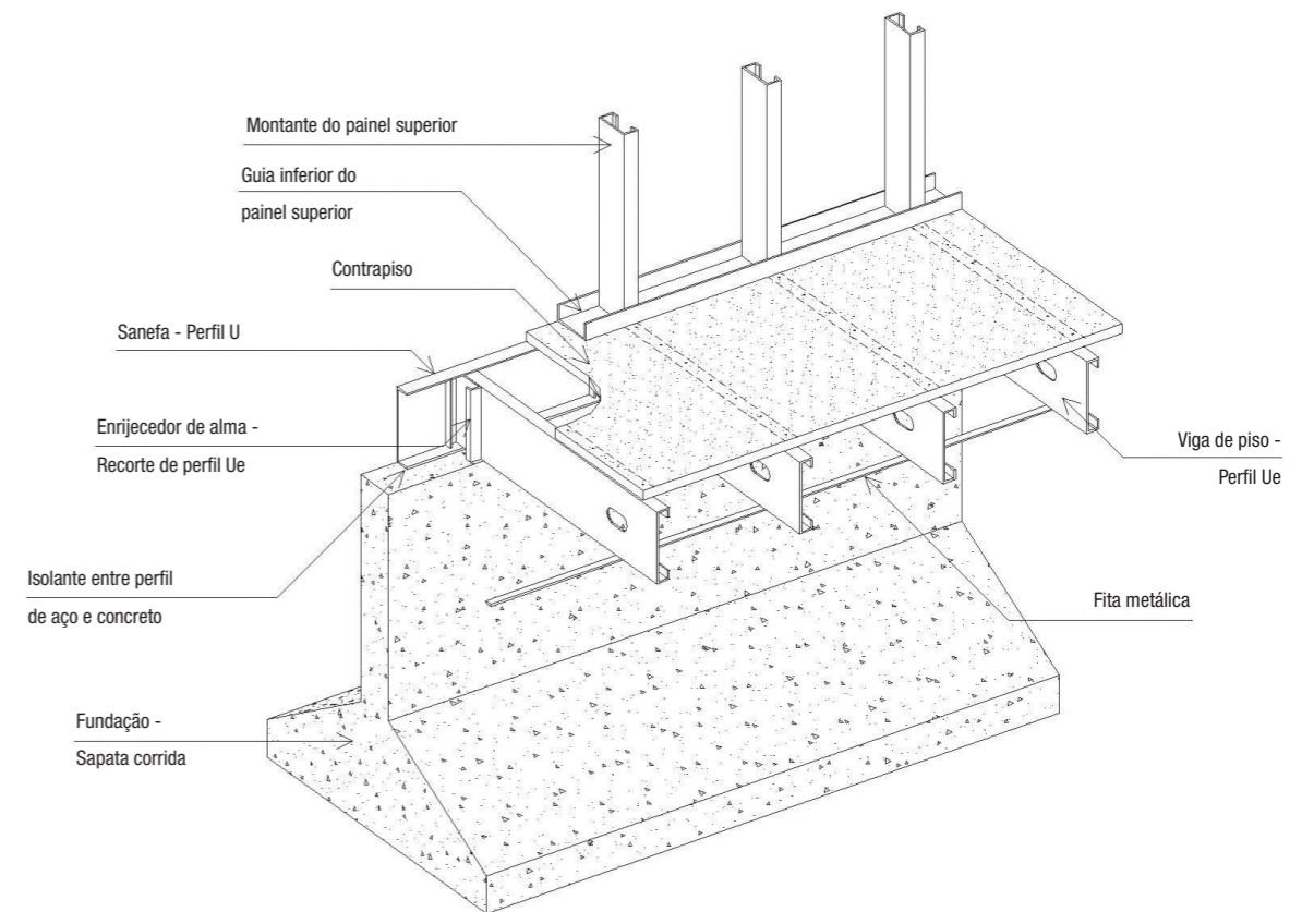
Figura 4.6 - Laje em Light Steel Framing apoiada sobre fundação tipo sapata corrida
