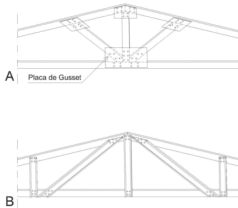
Figura 5.18 - Detalhe de cumeeira com tesoura (a) Howe e (b) Pratt
