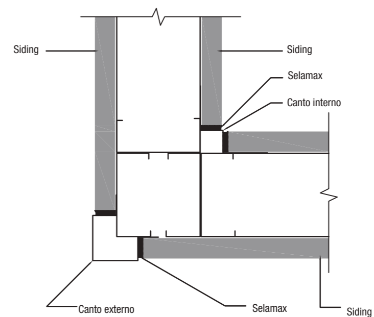
CORTE CANTOS COM PERFIS METÁLICOS
