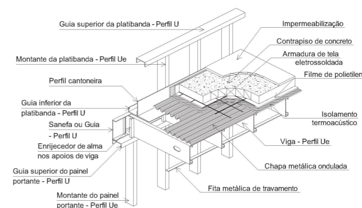
Figura 5.1 - Cobertura plana em Light Steel Framing
