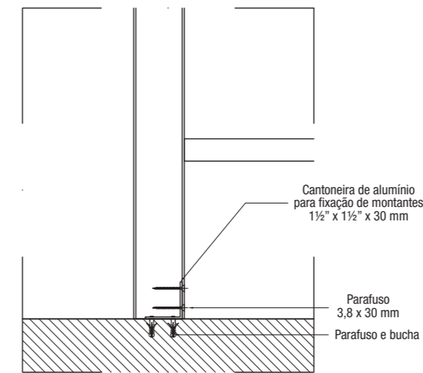
DETALHE 2
