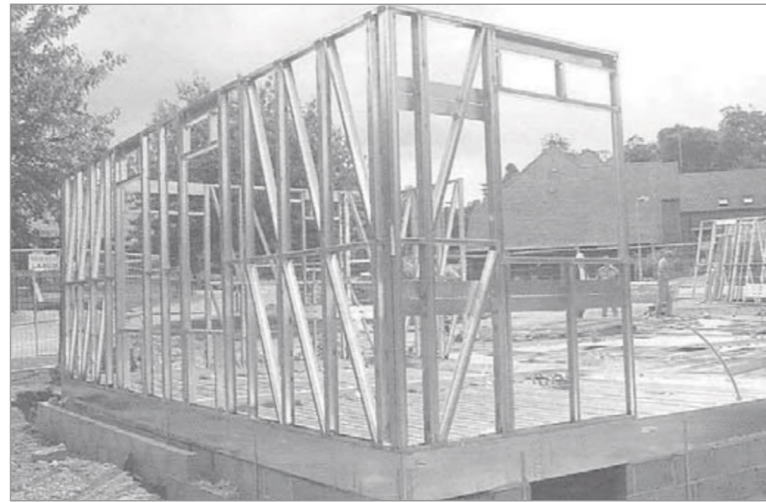
Foto 3.5 - Contraventamento em "K" (Fonte: SCI)
