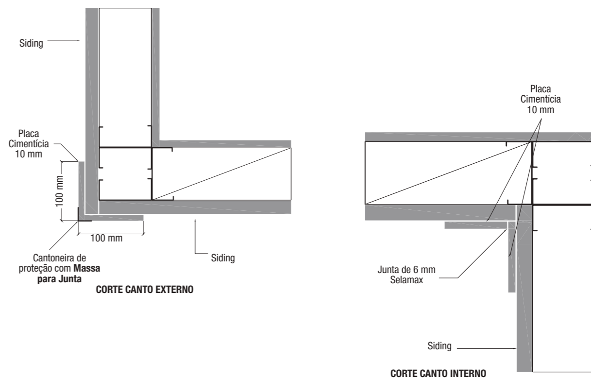
CORTE CANTO INTERNO
