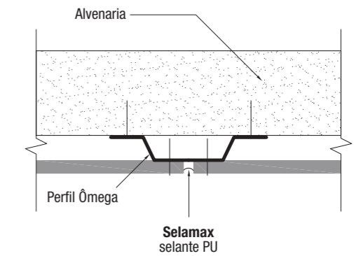
CORTE H-H
