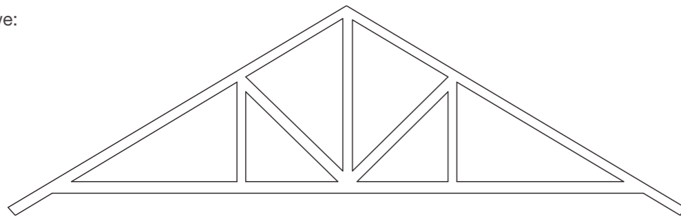
Figura 5.9 - Tesoura Howe
