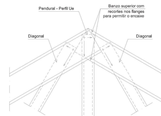
Figura 5.17 - Detalhe da cumeeira de tesoura Pratt
