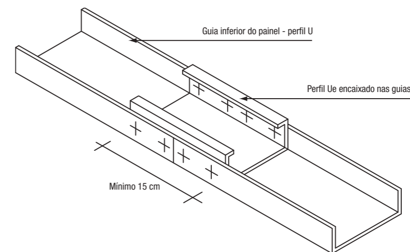
Figura 3.20 - Emenda de perfil guia
