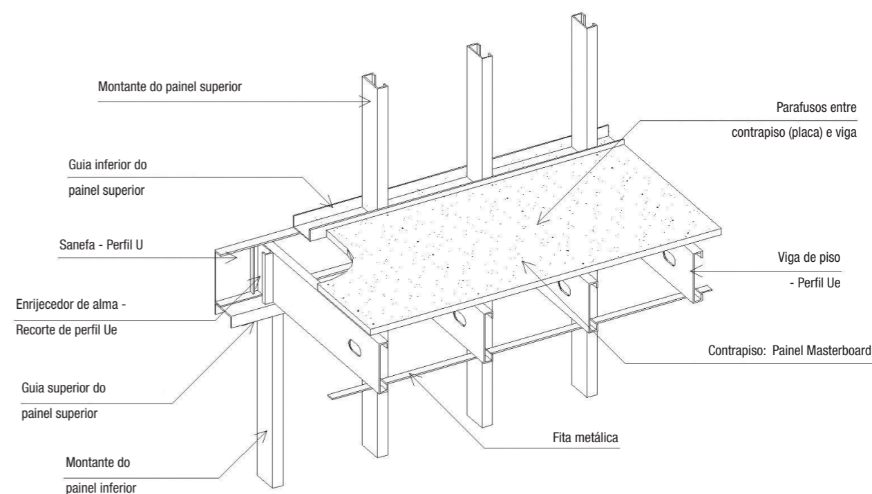
Figura 4.4 - Desenho esquemático de laje seca com painel Masterboard
