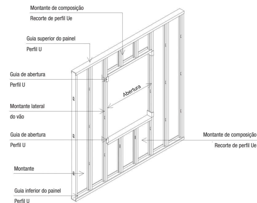
Figura 3.21 - Desenho esquemático de painel não estrutural com abertura
