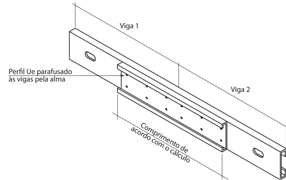
Figura 4.13 - Emenda de viga de piso
