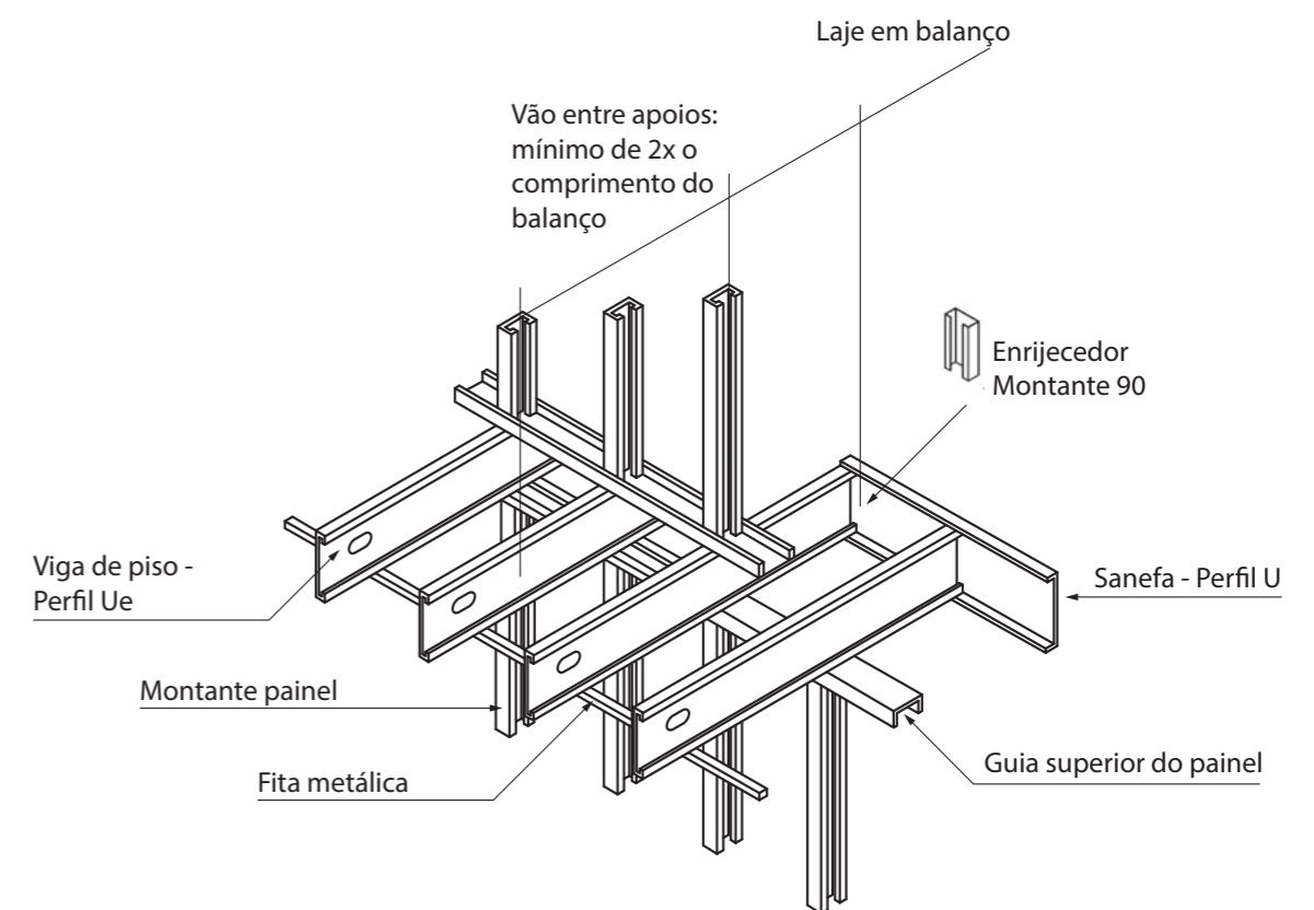
Figura 4.7 - Laje em balanço
