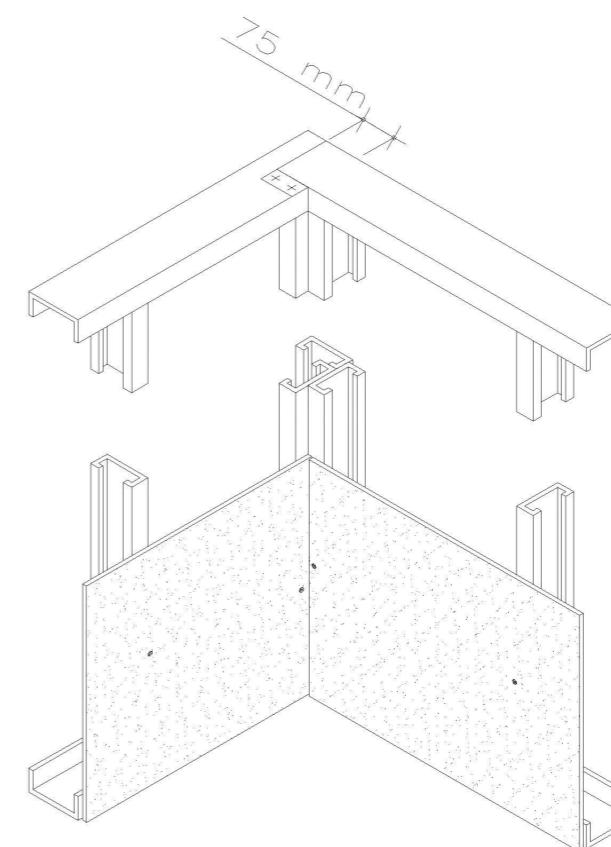
Figura 3.17 - Fixação de painéis de canto
